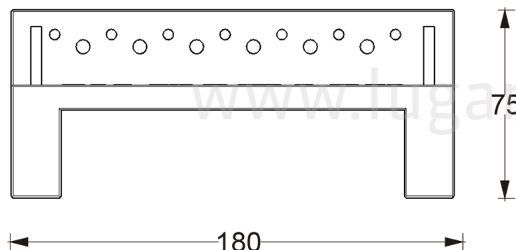
ELEVACIÓN FRONTAL
