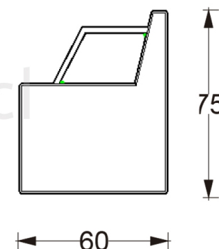
ELEVACIÓN LATERAL
